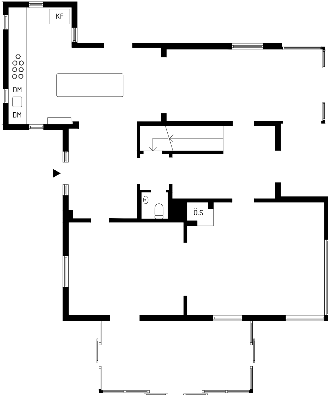
ENTRÉPLAN
